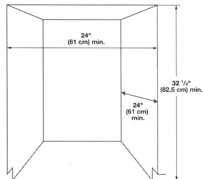
Cutout Dimensions
