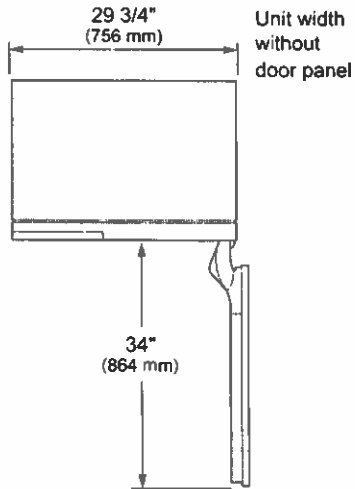
DOOR OPEN 90°
