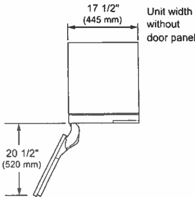
DOOR OPEN 115°
