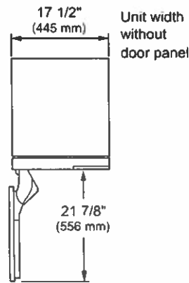
DOOR OPEN 90°
