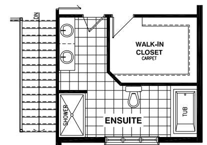
Optional 5 Pc Ensuite
