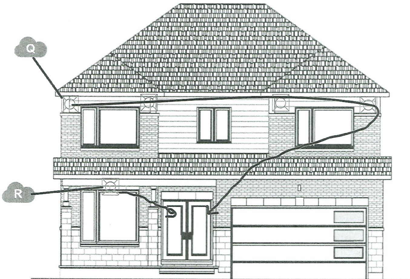
ELEVATION B
