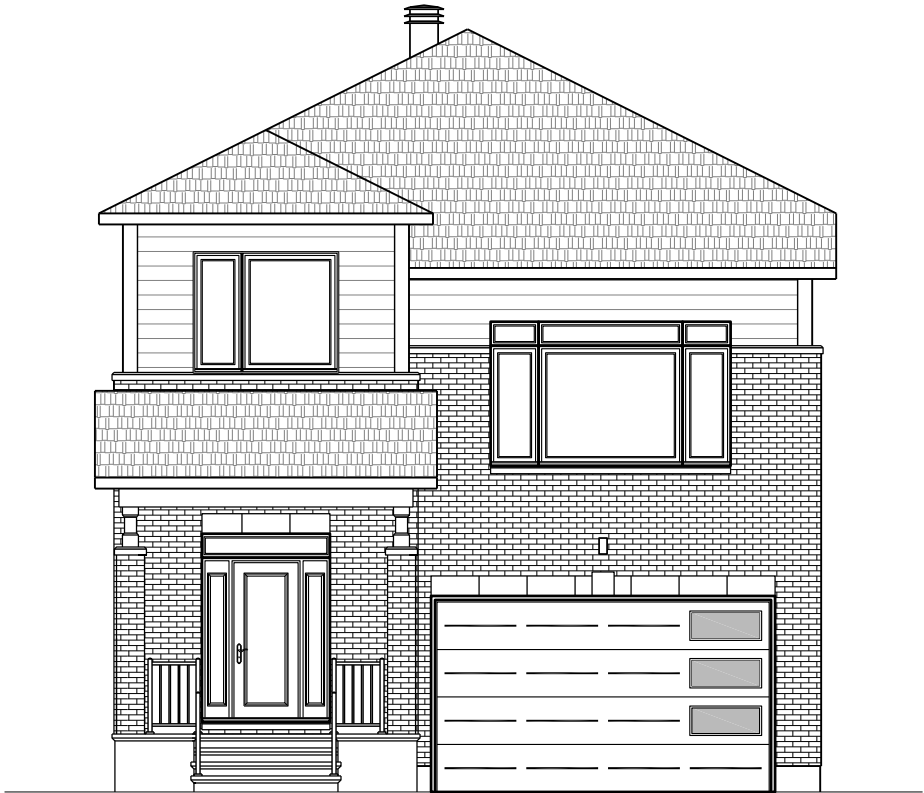
ELEVATION B
