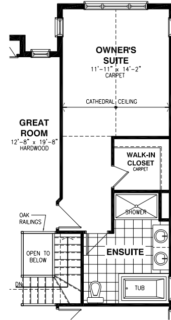
Optional 5 Pc Ensuite
