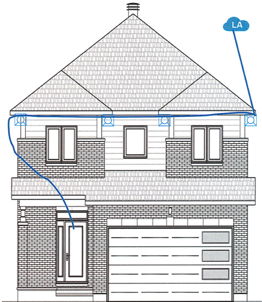
ELEVATION B
