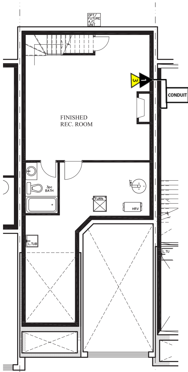
457.24 sq.ft. fin bsmt BASEMENT FLOOR
