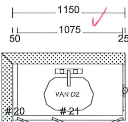
ENSUITE
