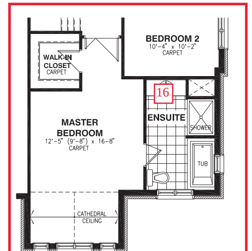
OPTIONAL 4 PC ENSUITE
