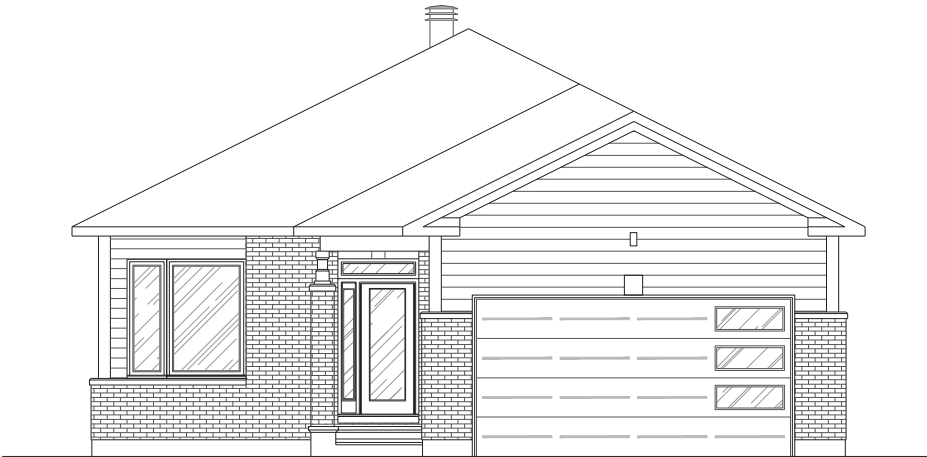
ELEVATION B
