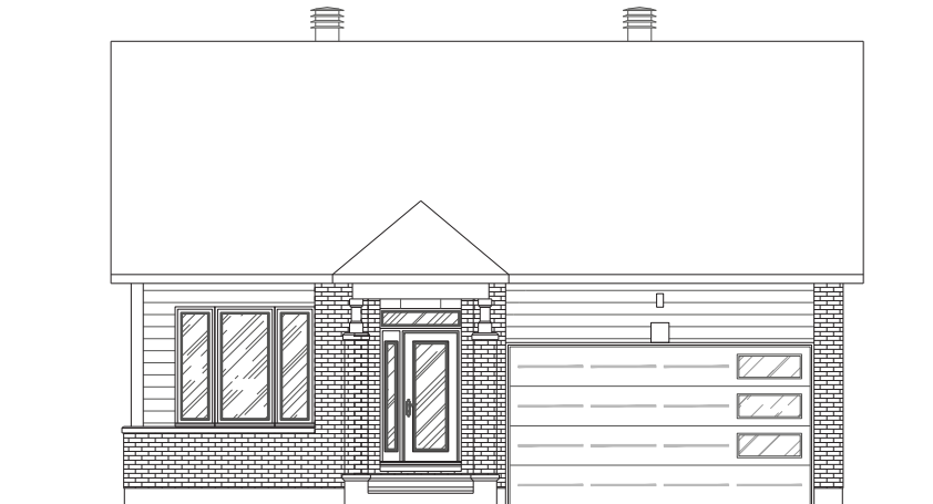
ELEVATION B
