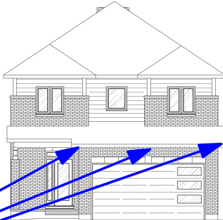
ELEVATION B
