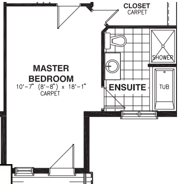
OPTIONAL 4PC ENSUITE BATH & SHOWER
