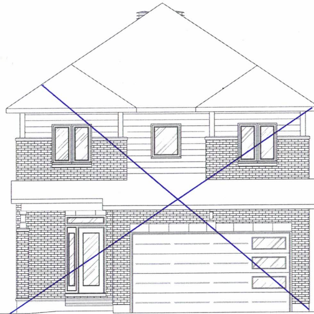
ELEVATION B
