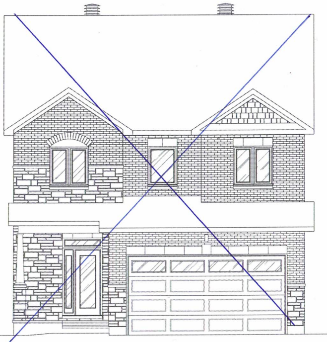
ELEVATION A
