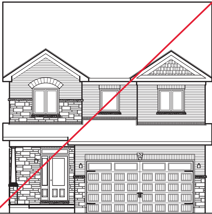
ELEVATION A
