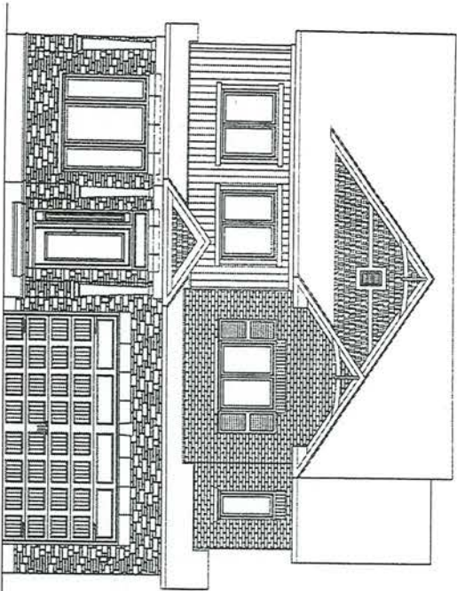
ELEVATION A
