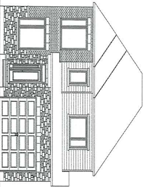
ELEVATION B
