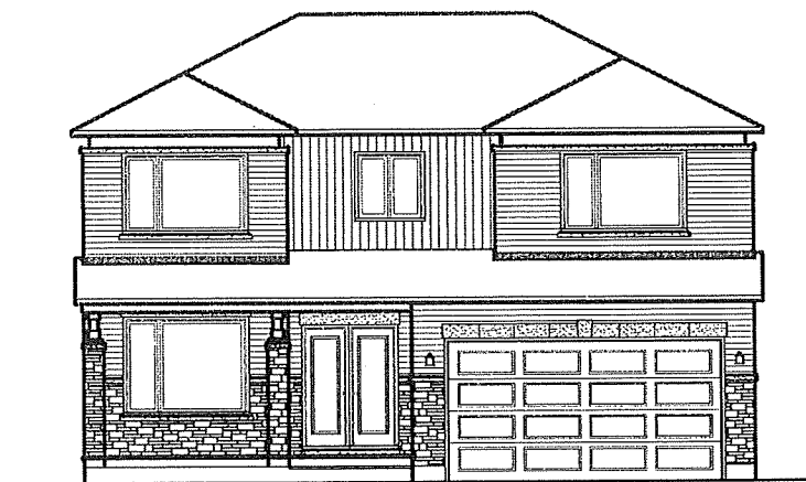
ELEVATION B
