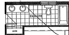
OPTIONAL 4PC ENSUITE
