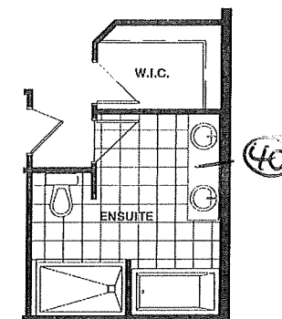
OPTIONAL 5PC ENSUITE
