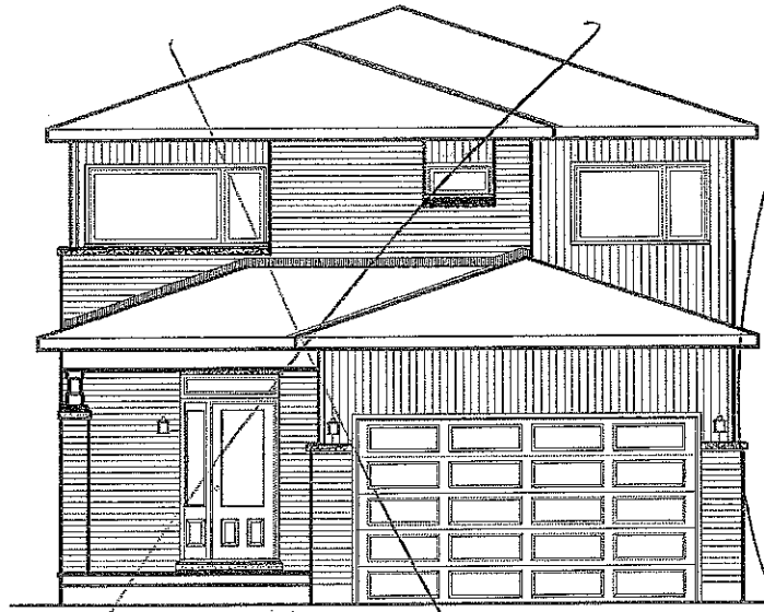
ELEVATION B
