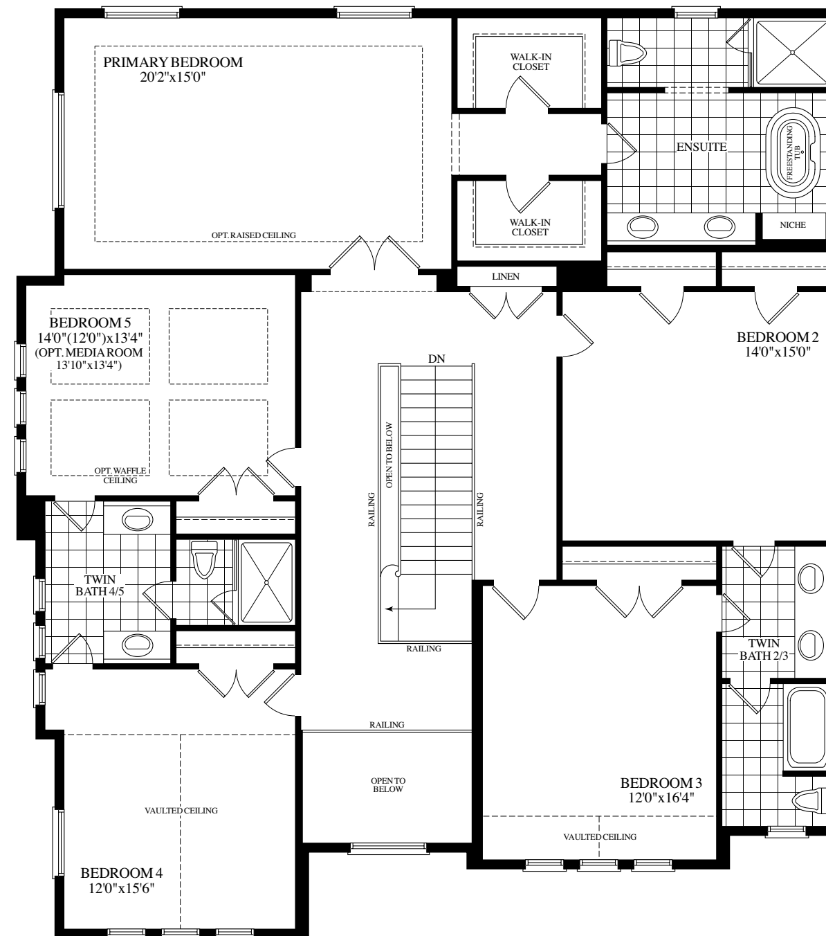
UPPER LEVEL ELEV.A
