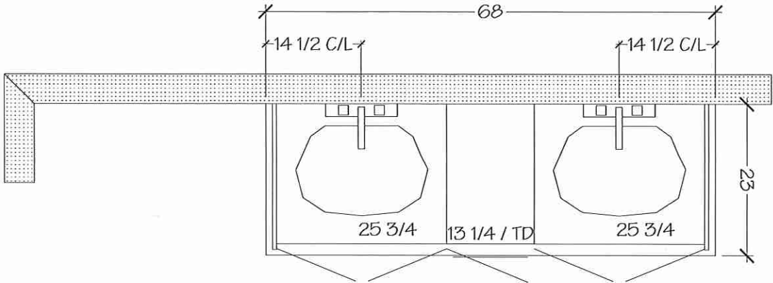
MASTER ENSUITE
