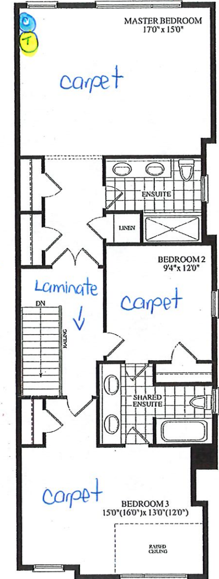
UPPER LEVEL ELEV.A
