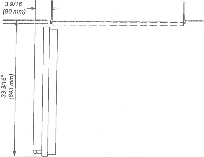
Door Swing
