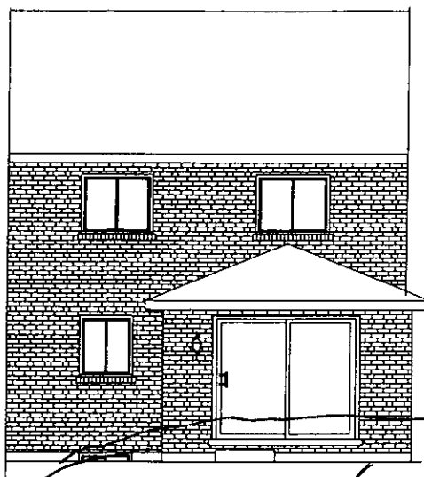
Back Elevation (WALK OUT)
