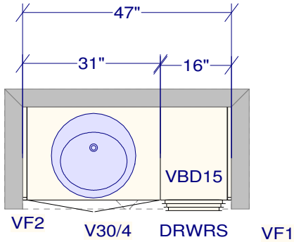
2ND. ENSUITE
