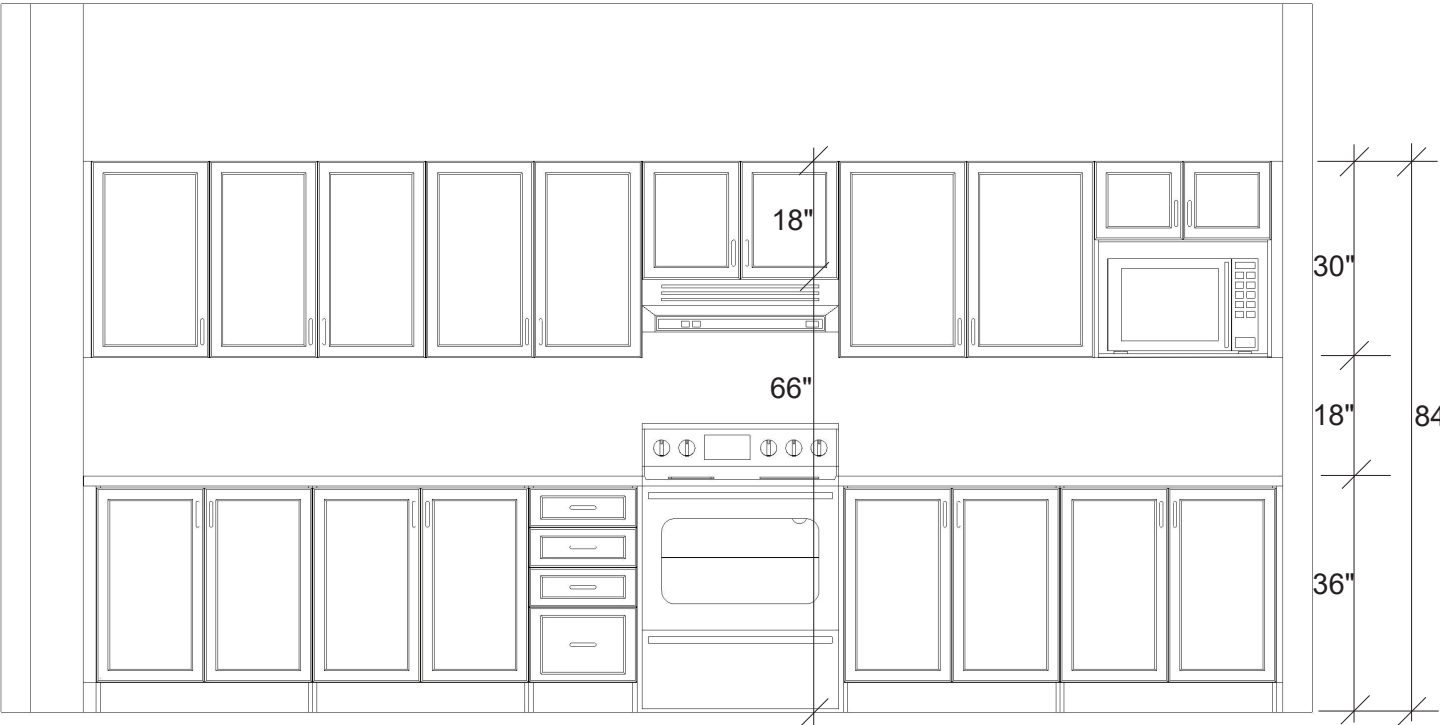
RANGE ELEVATION
