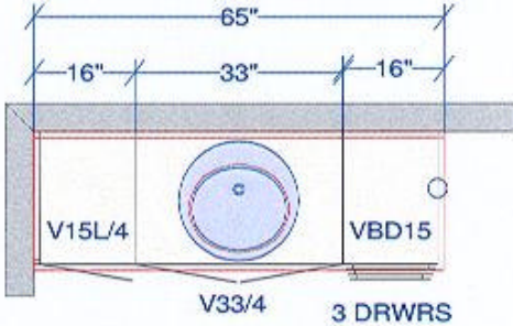
ENSUITE #2
