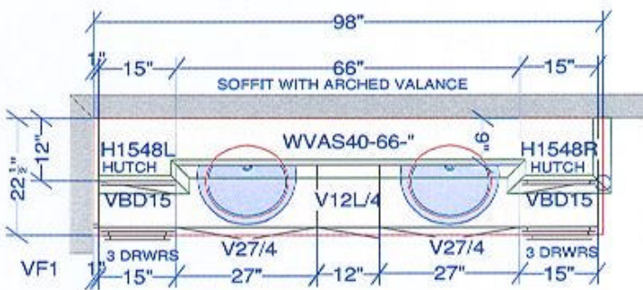
MASTER ENSUITE
