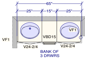
ENSUITE
