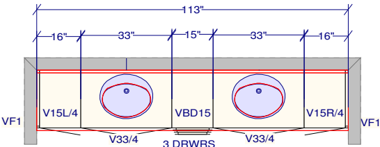
BEDROOM 3 & 5 - JACK & JILL ENSUITE
