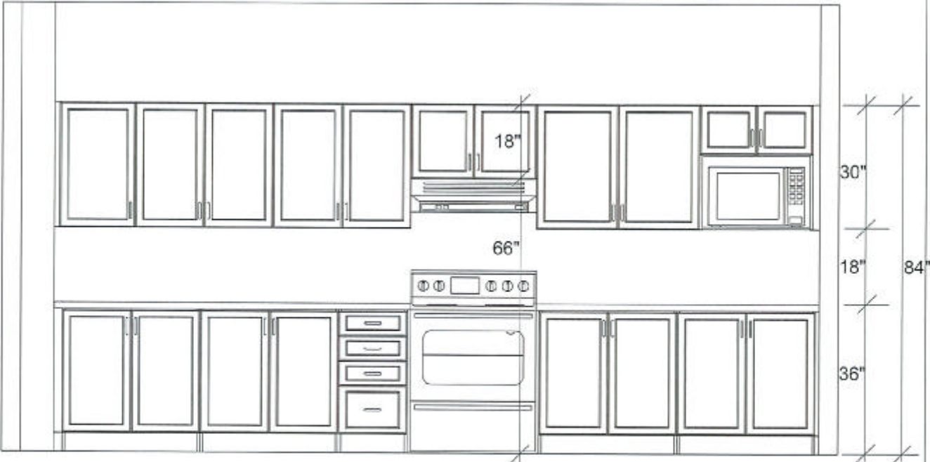
RANGE ELEVATION
