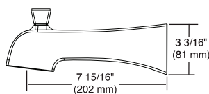
RP77091▲ (Pull-Up Diverter)
