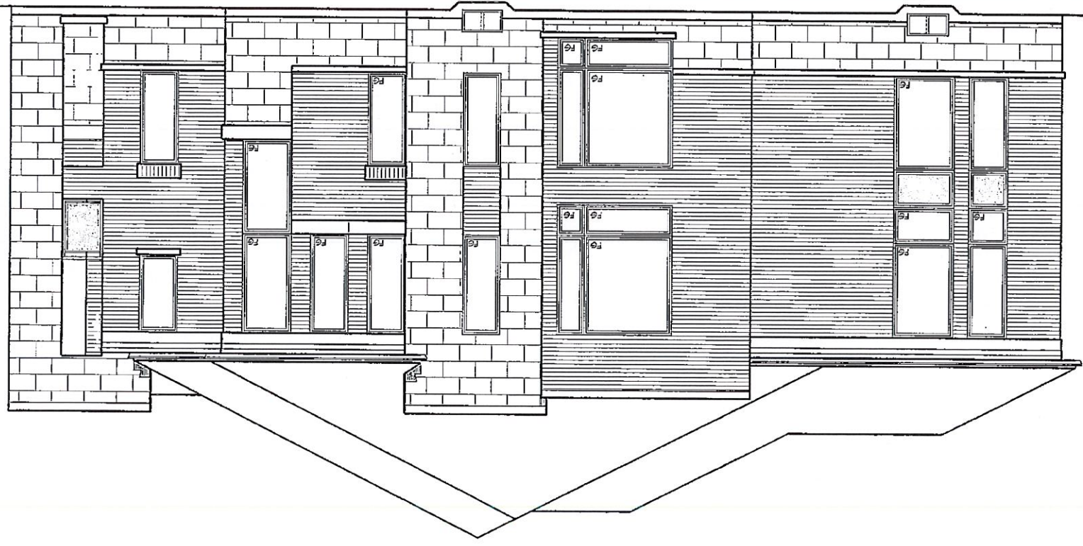
FLANKAGE ELEVATION
