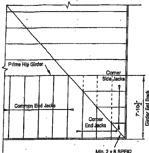
45° Hip End
