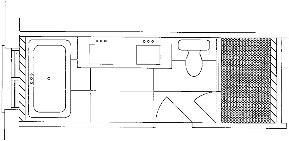
TM-16-4 PRINCIPAL ENSUITE PLAN
