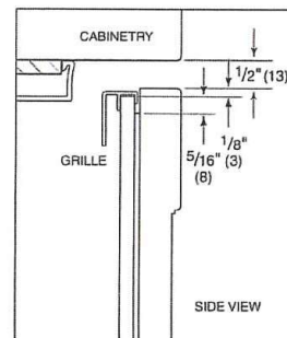
Grille Top
