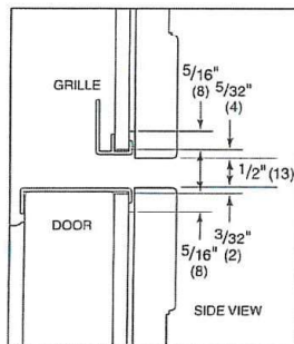
Grille Bottom / Door Top
