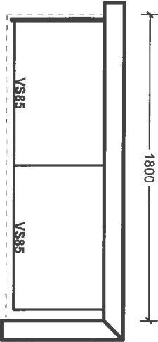
ENSUITE OPT 2 SINKS
