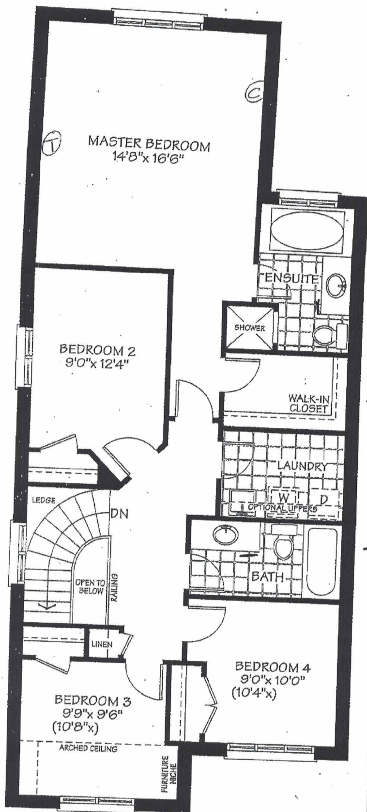
ELEV - B
