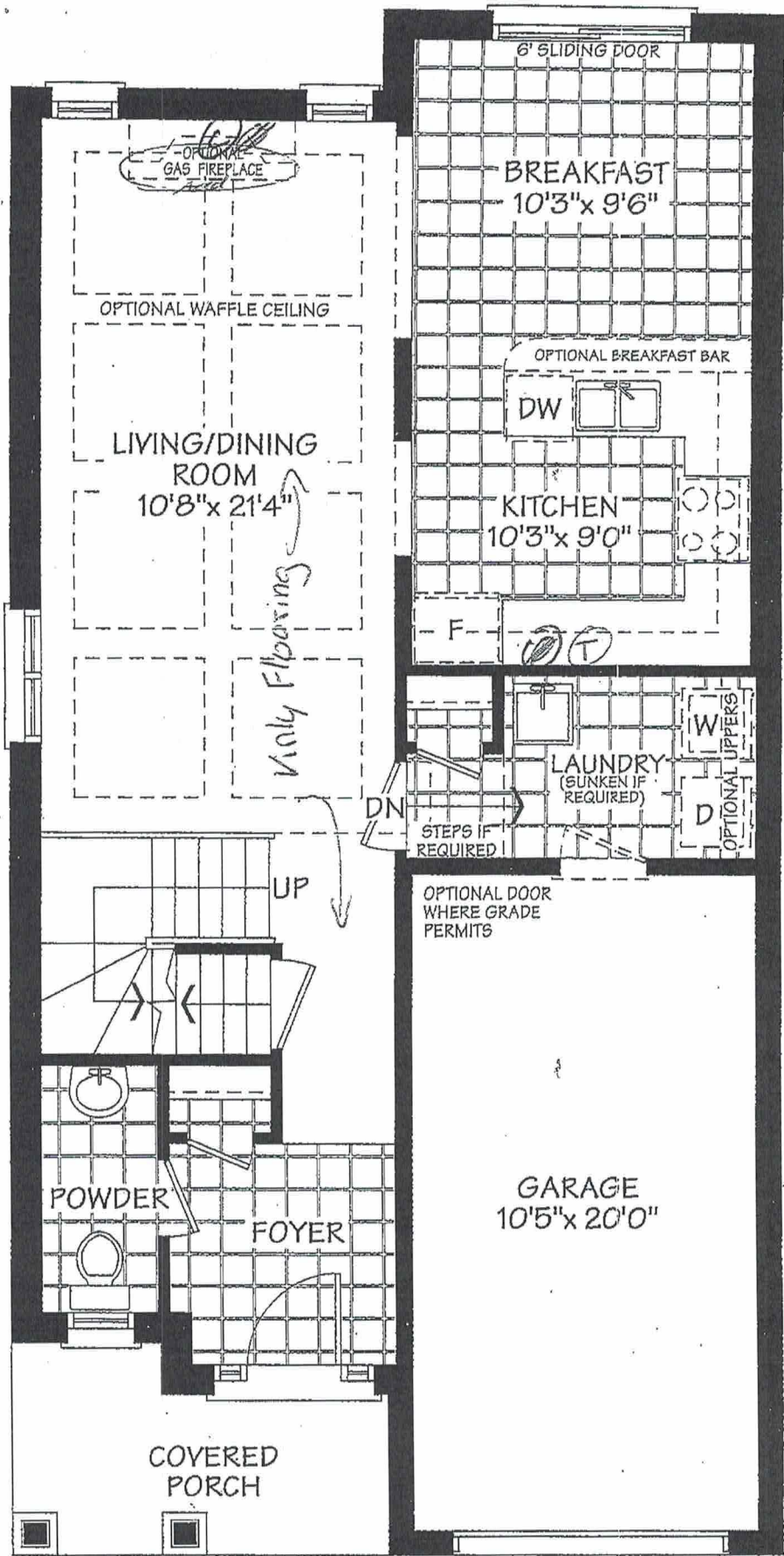
ELEV - B
