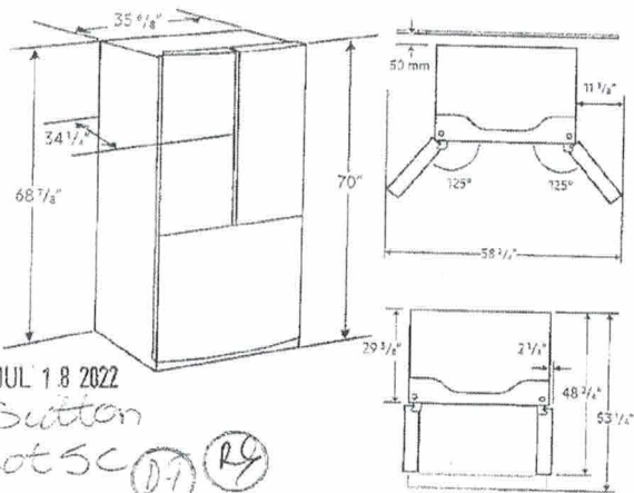
Dimensions
